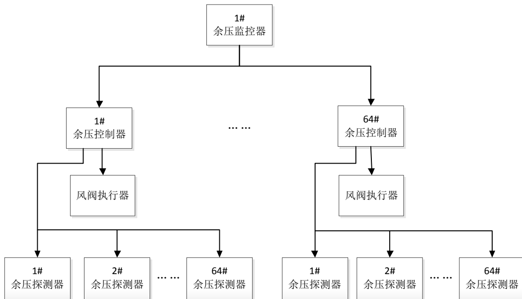
消防应急疏散余压监控系统示意图
