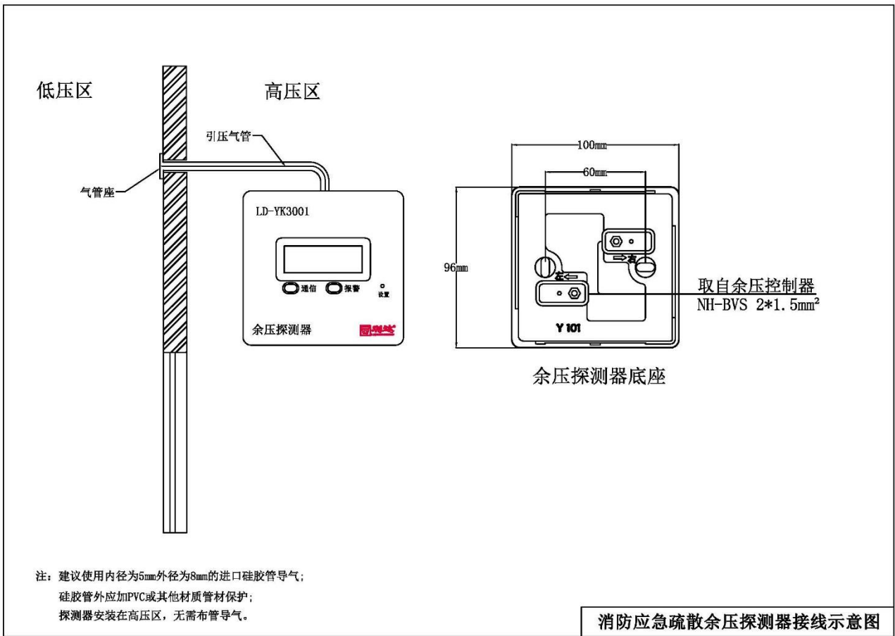
探测器接线示意图
