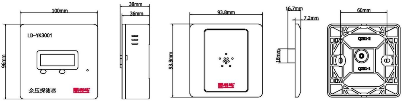
探测器安装尺寸及安装孔位示意图
